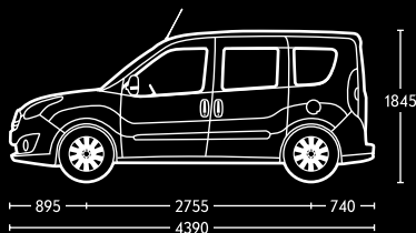
Combo Cargo L1H1 avec portes latérales vitrées.
