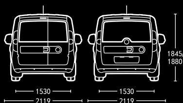
Combo Cargo avec portes arrière asymétriques ou hayon.
