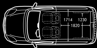
Combo Cargo L1H1 ou L1H2.
