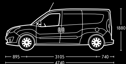
Combo Cargo L2H1.
