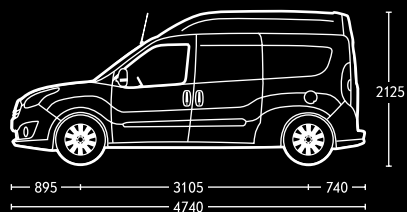
Combo Cargo L2H2.
