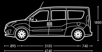
Combo Cargo L2H1 avec portes latérales vitrées.
