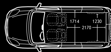
Combo Cargo L2H1.
