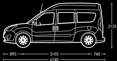
Combo Cargo L2H2 avec portes latérales vitrées.
