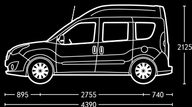
Combo Cargo L1H2 avec portes latérales vitrées.
