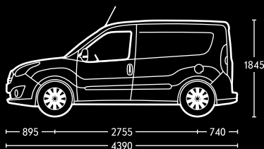
Combo Cargo L1H1.
